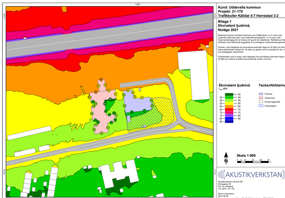
Figur 11. Ekvivalent ljudnivå i dag. Källa: Akustikverkstan, 2021-06-28
