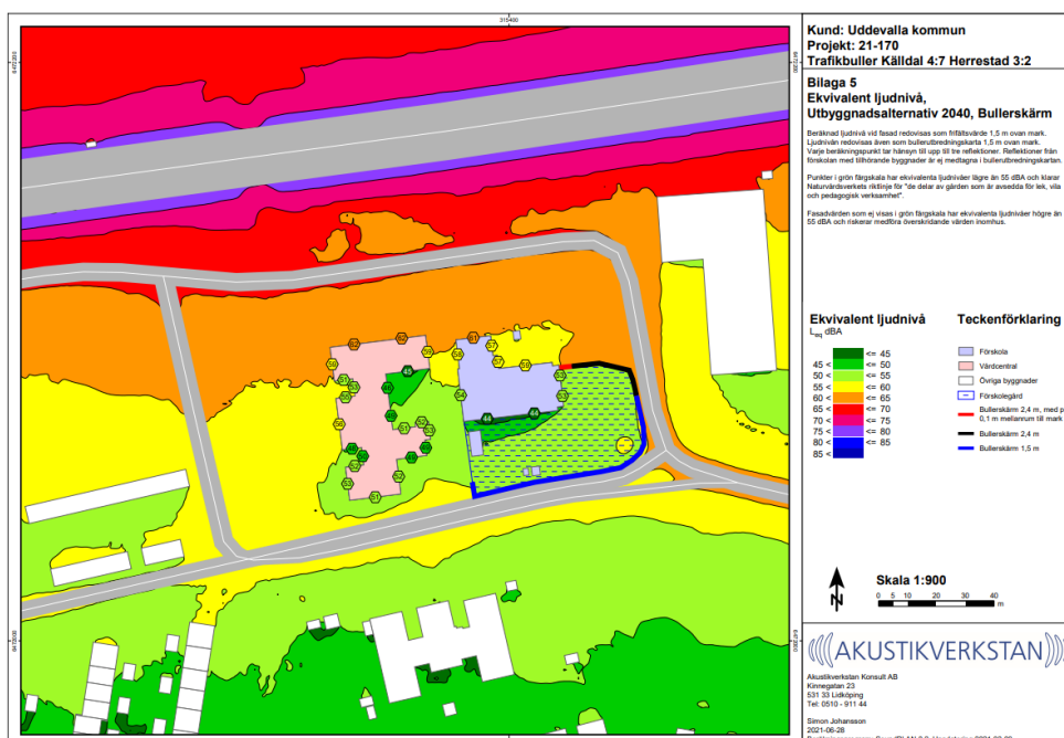
Figur 12. Utbyggnadsalternativ. Källa: Akustikverkstan, 2021-06-28
